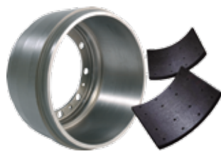
Тормозные барабаны и накладки
